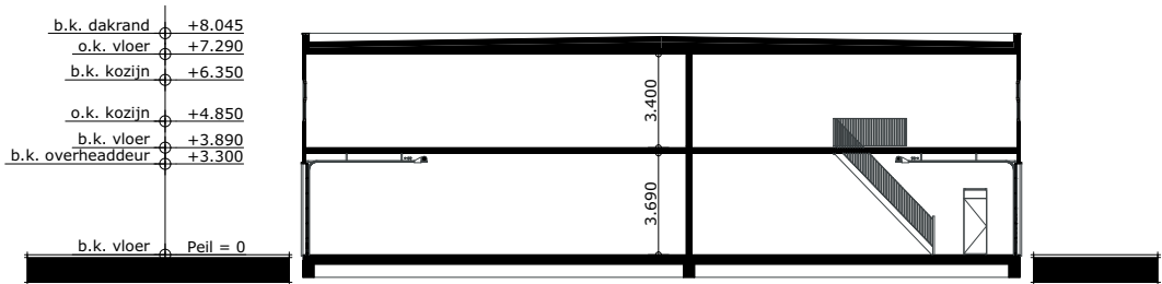
DOORSNEDE B-B
