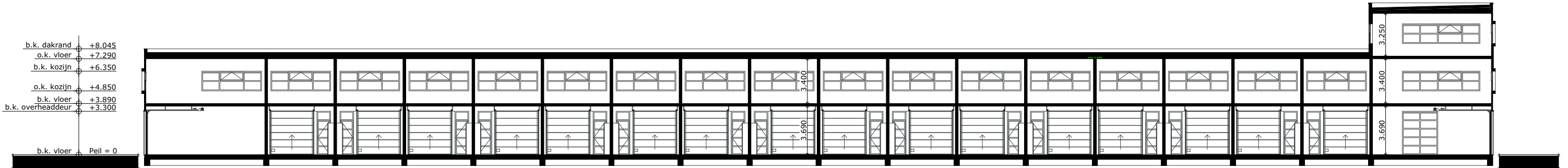
DOORSNEDE A-A
