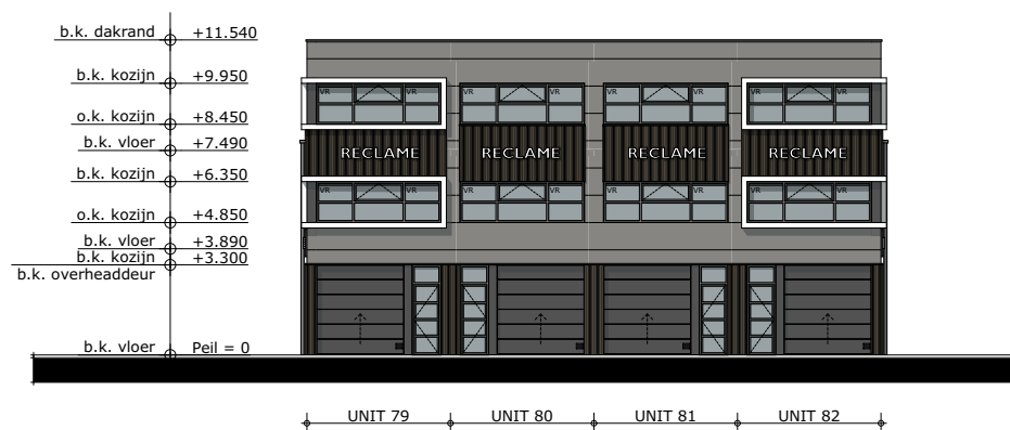
ZUID-OOST GEVEL
