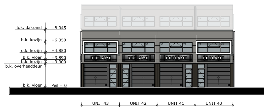
NOORD-WEST GEVEL
