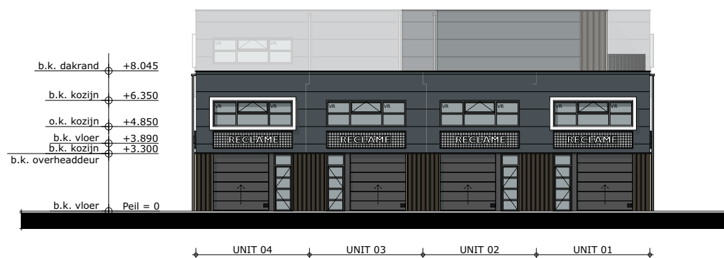
NOORD-WEST GEVEL
