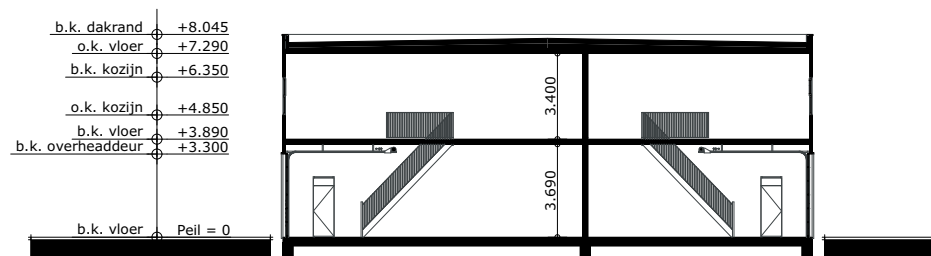
DOORSNEDE B-B
